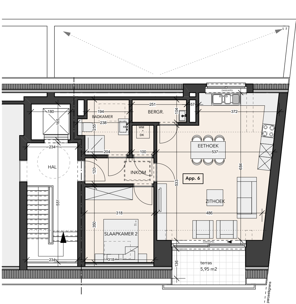
APPARTEMENT 6 - bruto opp.: 78,81 m 2
