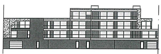
VOORGEVEL
