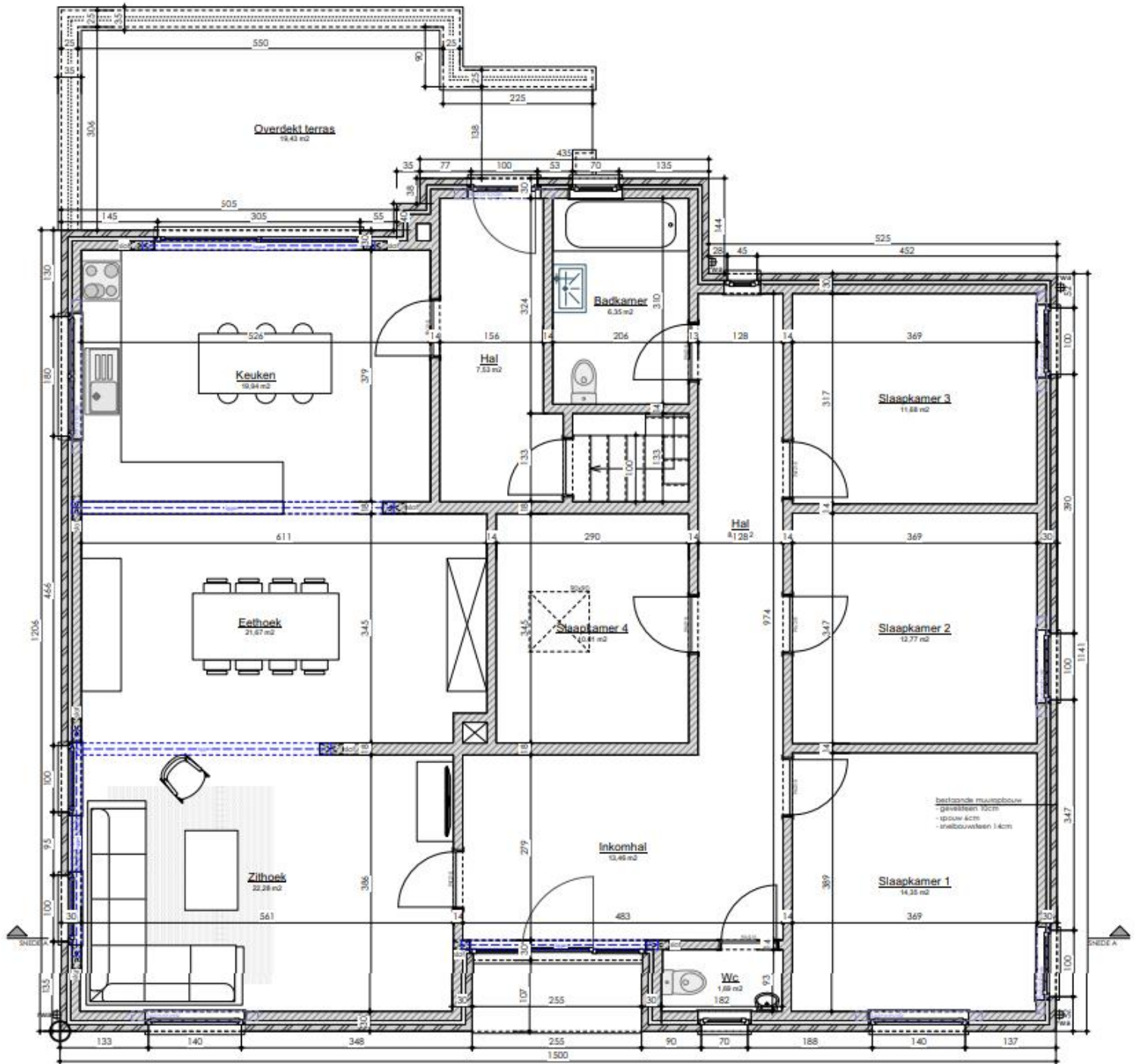
Grondplan - Bestaande toestand Schaal: 1:50
