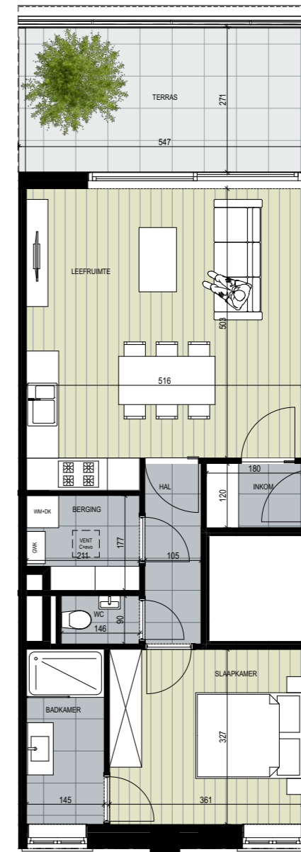
Niveau +1
