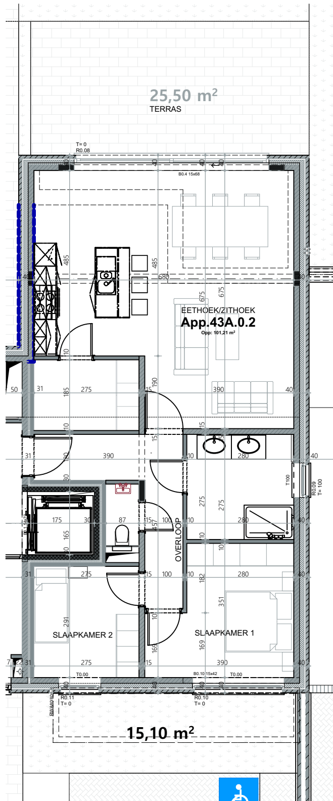
0. Appartement 43A.0.2 1:100
