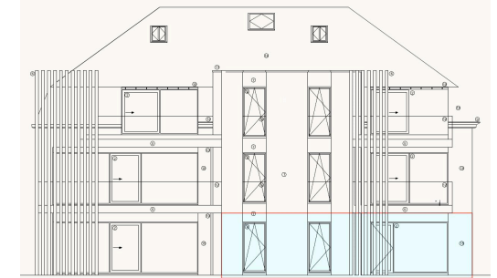
ACHTERGEVEL (NW)
