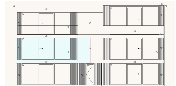
VOORGEVEL (ZW)
