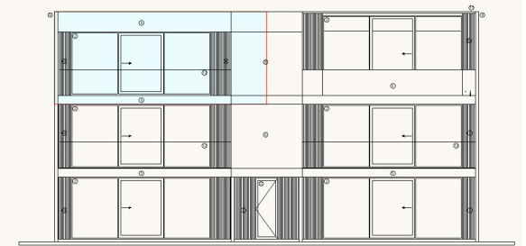
VOORGEVEL (ZW)
