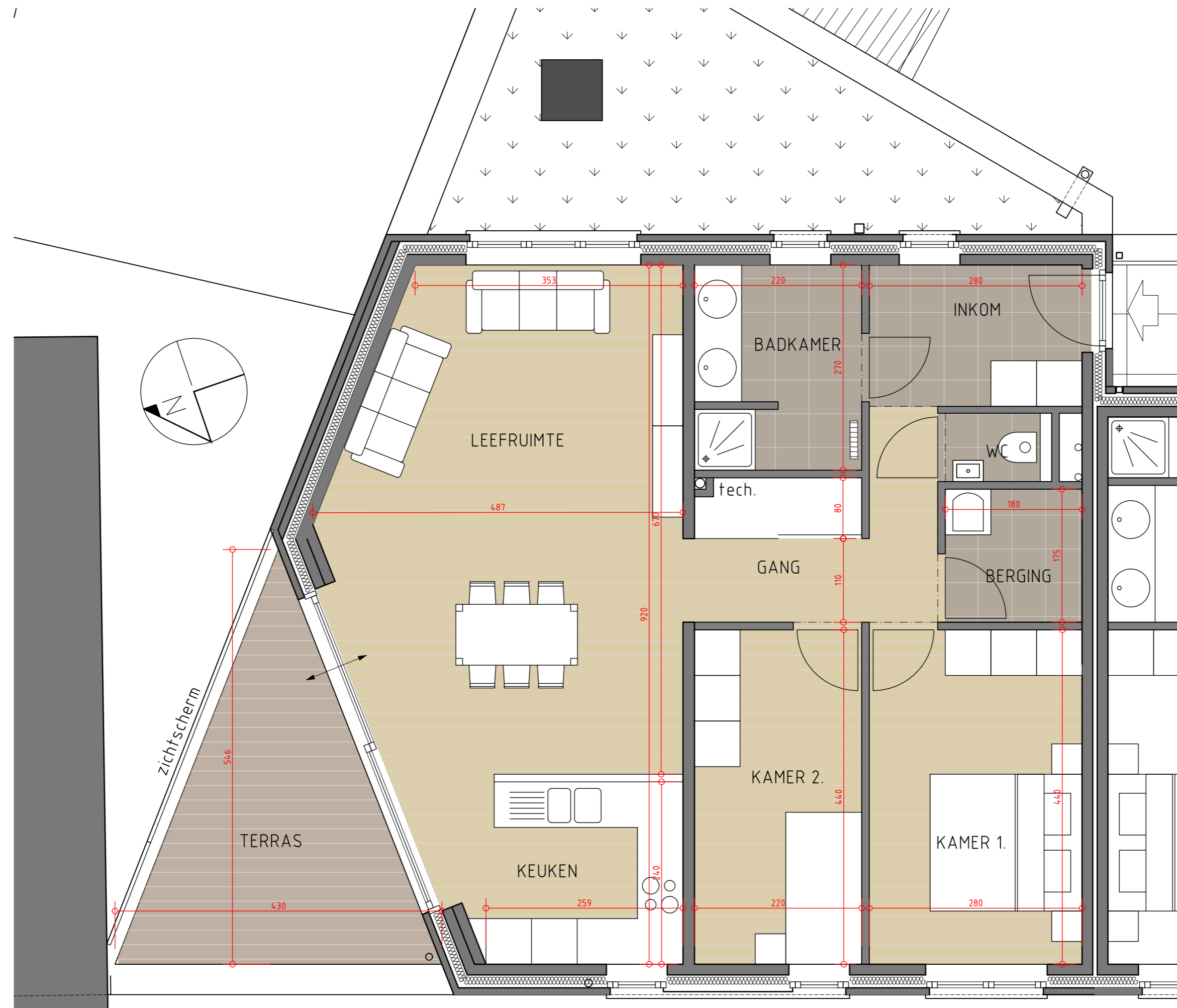
VERDIEPING 1 : APPARTEMENT 5
