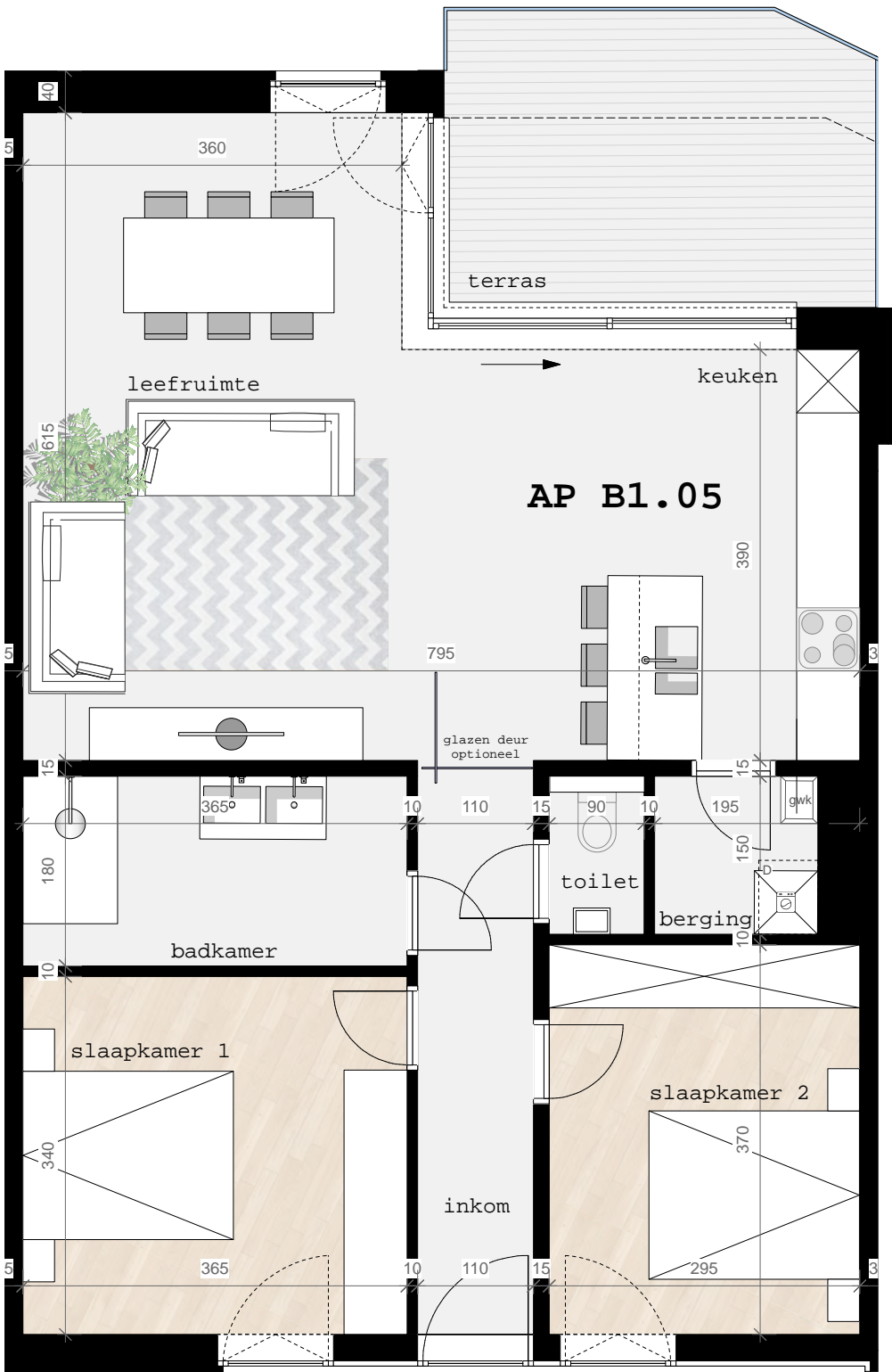
Grondplan
