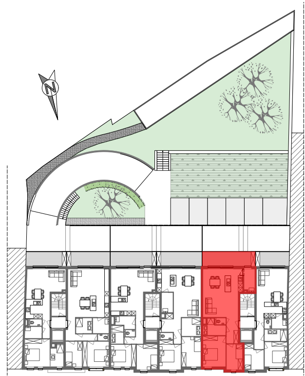
GRONDPLAN EERSTE VERDIEPING
