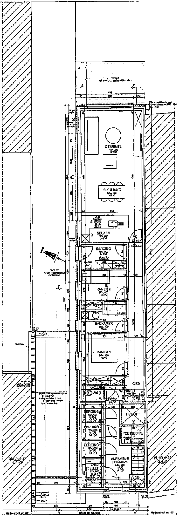
GELIJKVLOERS Reëntal 000 = L.12.00 H. (duitsmaat) 207cm (tent) onder vermeld to 200 G 1 2 3 4 5m
